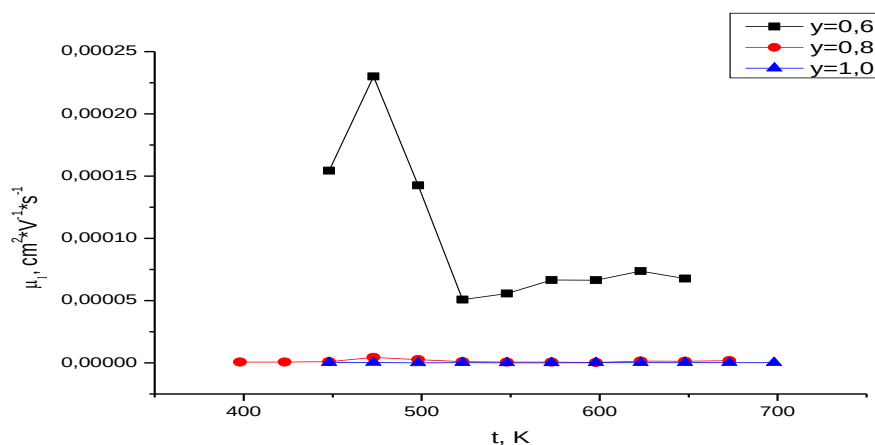
Рис. 1. Залежність макроскопічної рухливості \mu_1 катіонів літію від температури при різних значеннях вмісту алюмінію в синтезованих зразках
