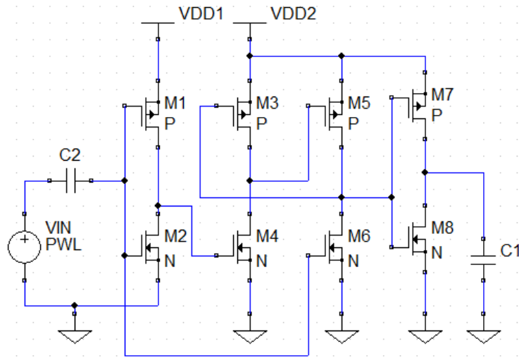
Рис. 1. Базова електрична схема для дослідження і оцінювання ємностей ССЕ в МнК на основі КМОН транзисторів
