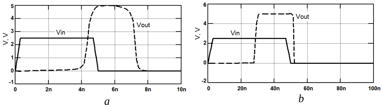
Рис. 2. Форми входних і вихідних сигналів схем з підключеним ССЕ: а – T_{in}=10 ns; б – T_{in}=100 ns
