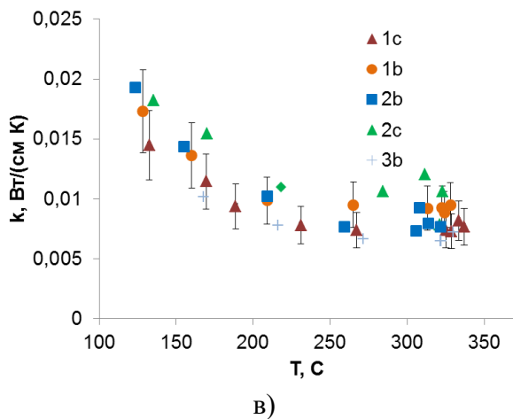
Рис. 1. Температурна залежність питомої електропровідності \sigma (а), коефіцієнта термо-ЕРС \alpha (б) та коефіцієнта теплопровідності k (в) зразків (\text{Pb}_{0.6}\text{Sn}_{0.4})_{0.9}\text{Cd}_{0.1}\text{Te} (Зразки 1a, 1b, 1c, 3a, 3b отримані при тиску пресування 1 ГПа, 2a, 2b, 2c – при тиску 0,75 ГПа).
