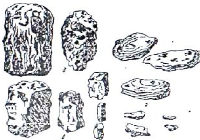
Рис.2. Формування структурних агрегатів: а - зерниста; б - горіхоподібна; в - призматична; г - шарувата; д - брилиста.
