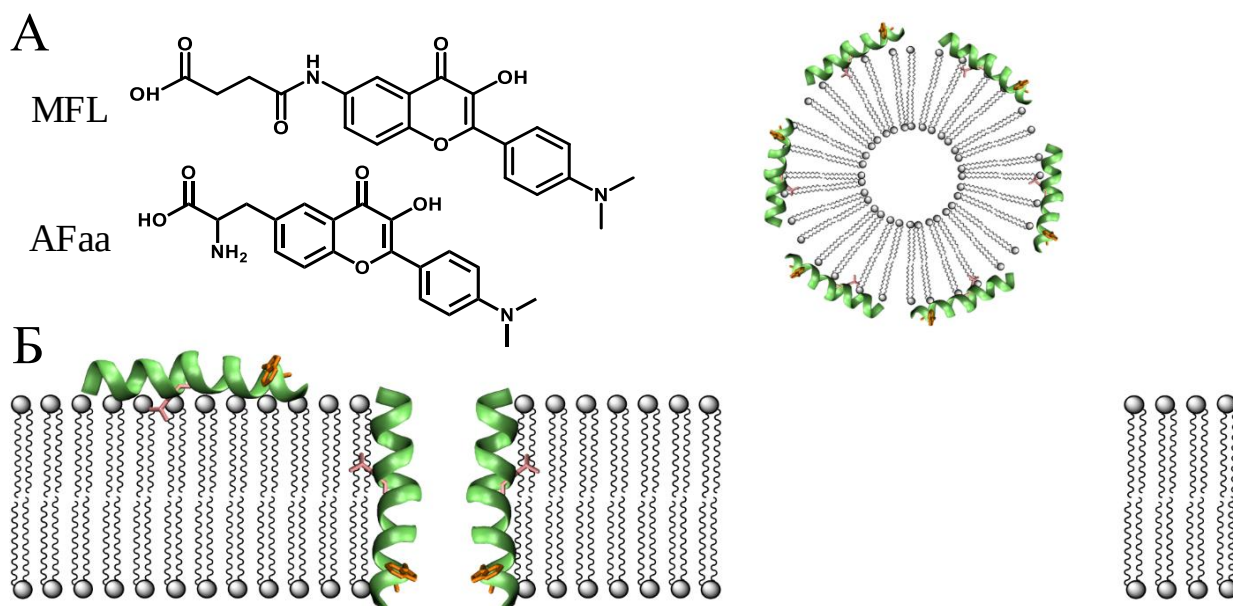
Рис. 1. А – Структура флуоресцентних міток. Мітка AFaa синтезована на основі тирозину та похідного 3-гідроксифлавоу. Б – Положення мелітину в мембрані.
